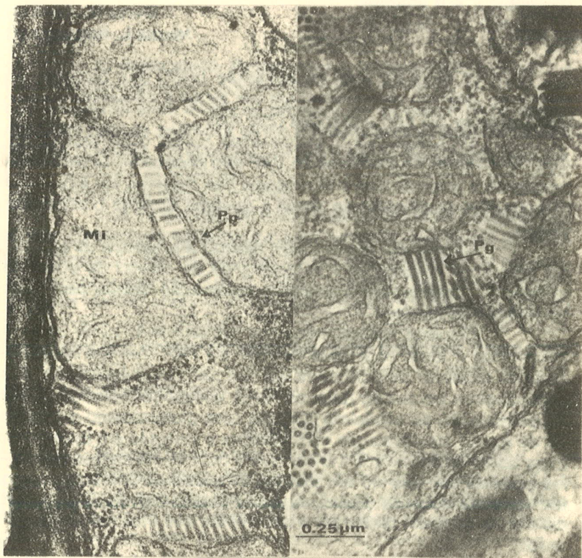
Eletrófotomicrografia de tecido foliar de fumo mostrando as partículas pequenas do Vírus do Anel do Pimentão. Pp - partículas pequenas; Pg - partículas infetivas; MI - mitocôndrio.
